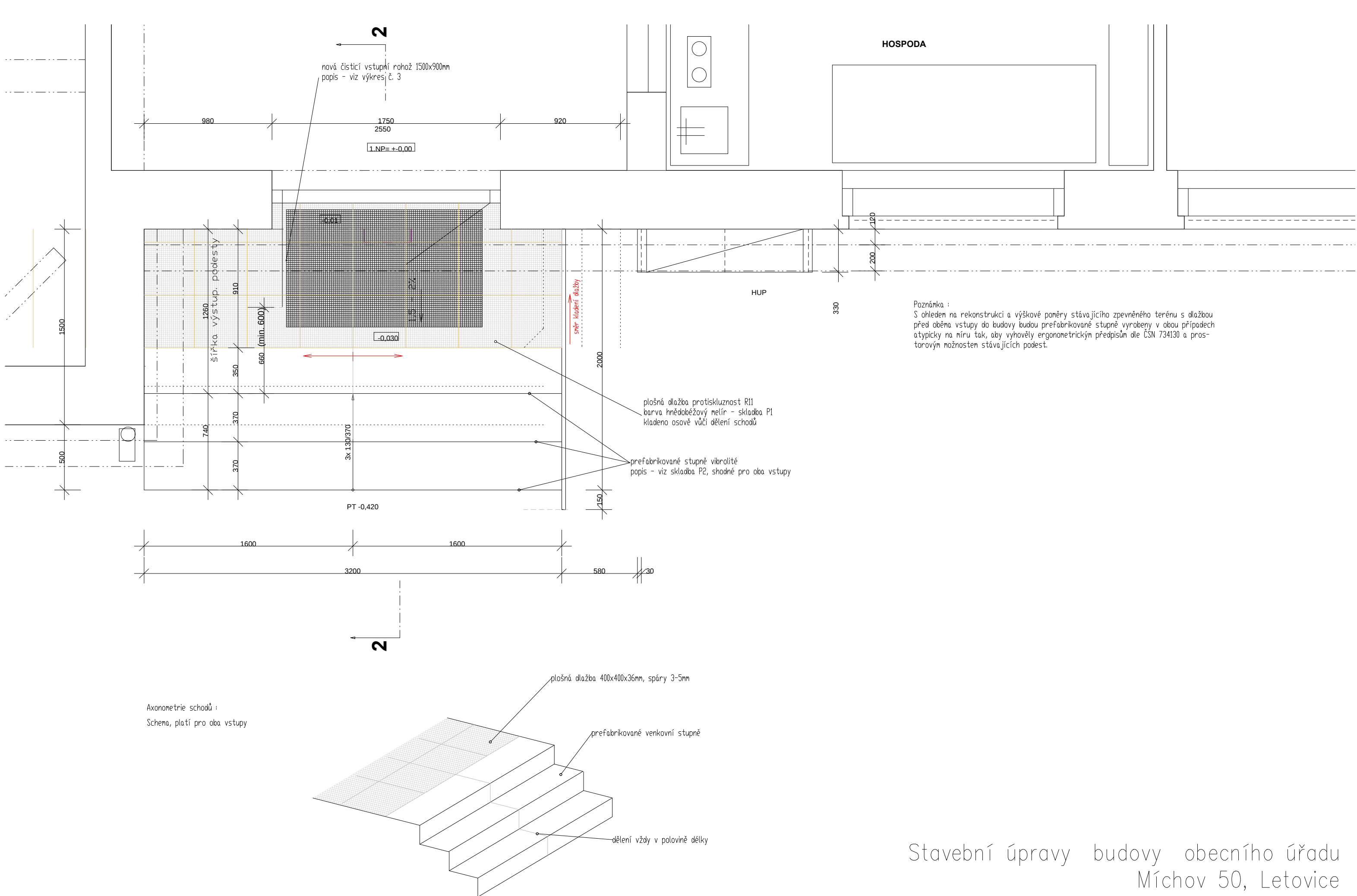
PŮDORYS 1.NP - Návrh vchod hospoda - výřez M 1:25
